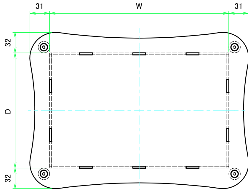
上カバー / Top cover
